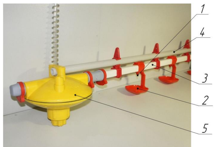
Рис. 1.6. Лінія напування птахів з ніпельною системою: 1 –ніпель; 2 – каплеуловлювач, 3 – трубопровод живильний; 4 – штанга, 5 – регулятор тиску.
